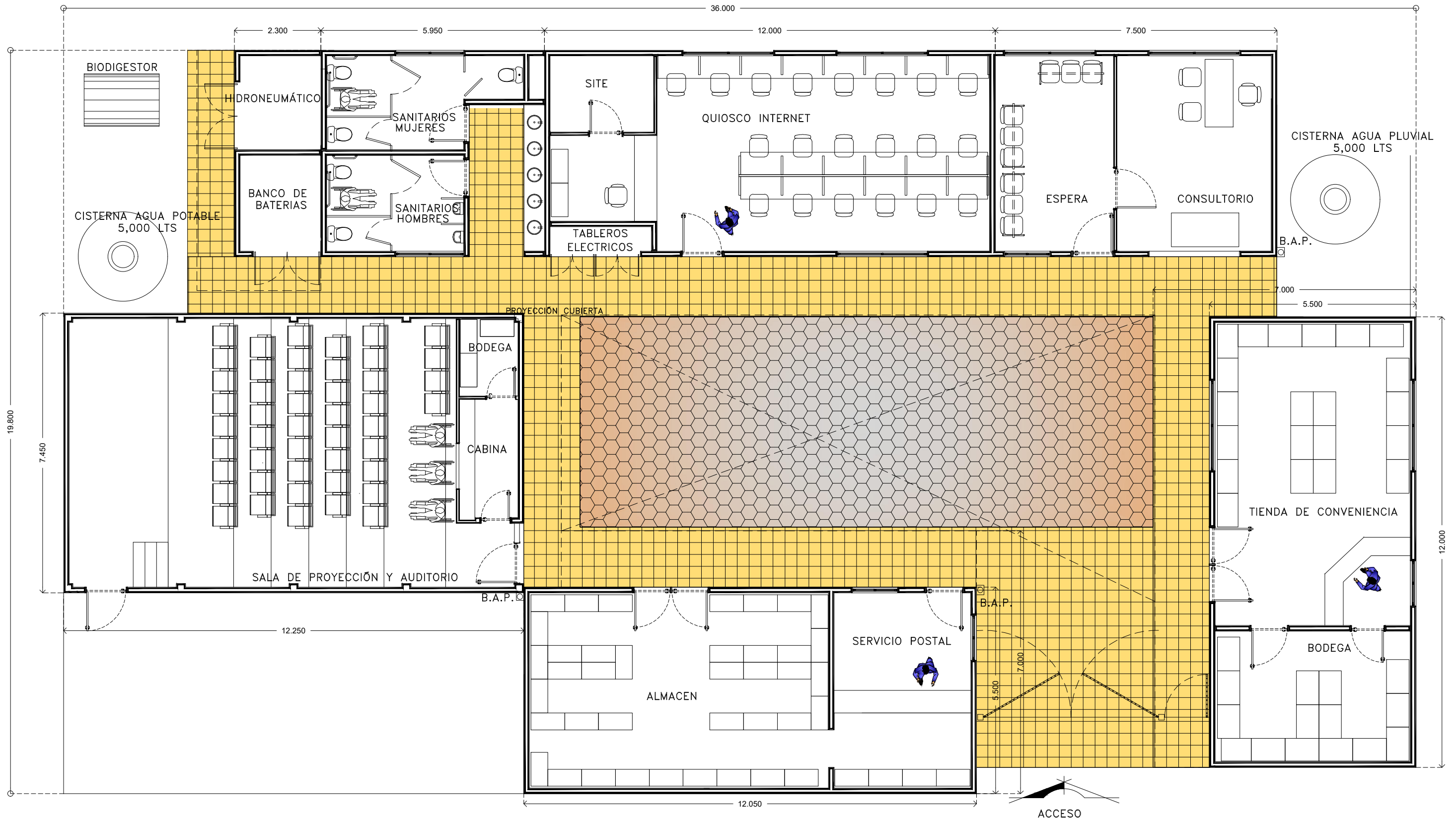
PLANTA BAJA CONSTRUCCION 463.87 M2
